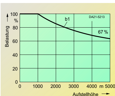
Kurve b1: Reduktionsfaktor der Belastungswerte (Gleichstrom) bei Aufstellhöhe über 1000 m
