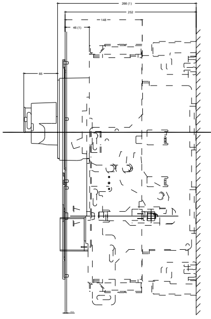
(1) Betriebsstellung (2) Trennstellung
