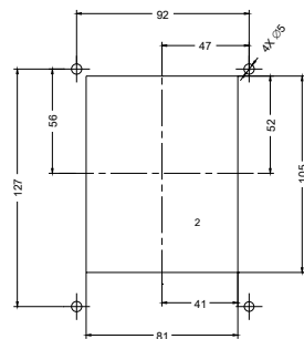
1 Türausschnitt Kipphebel ohne Blendrahmen 2 Türausschnitt Kipphebel mit Blendrahmen
