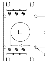
Bohrplan Tuer
