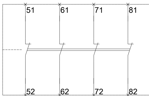
3RH2
