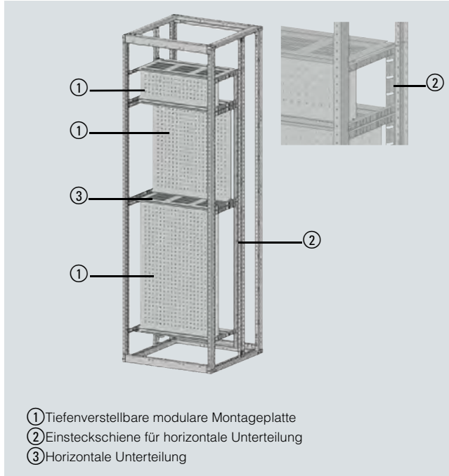
Modulare Montageplatten
