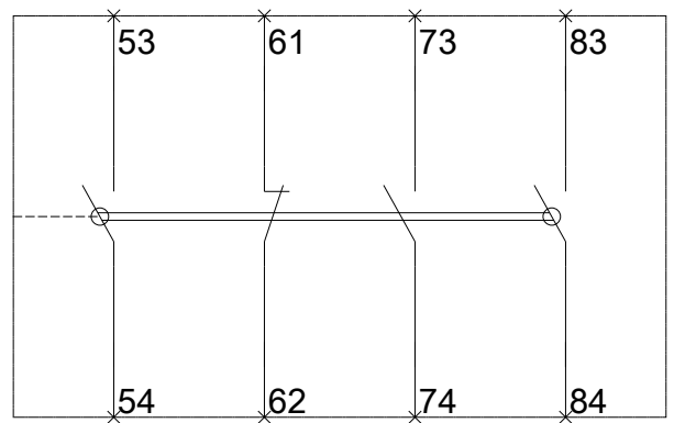
3RH2
