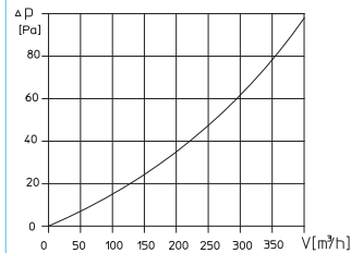
Druckverlust Außenluft-Ansaugsäule mit Filter G 3 und 40 Meter Erdkollktorrohr im Reinzustand
