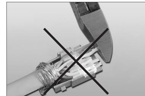
Mit einem ungeeigneten Seitenschneider lassen sich die Kabeladern nicht bündig abschneiden. Dies führt zu Problemen beim späteren Zusammenfügen der beiden Gehäuseteile. The wires cannot be cut really flush with an inappropriate wire cutter. Excess wire will cause problems when the two housing parts are assembled.
