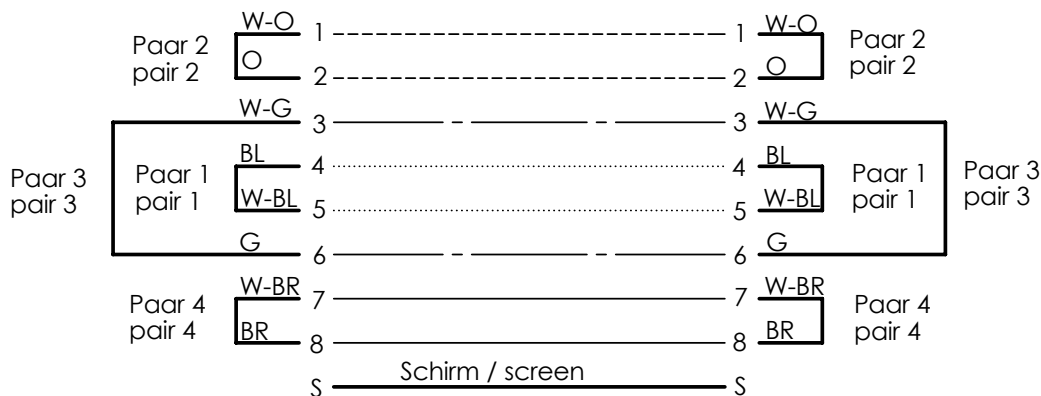
Stecker A plug A
