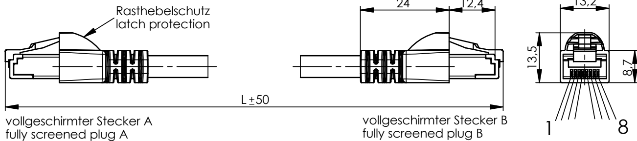
Stecker A plug A
