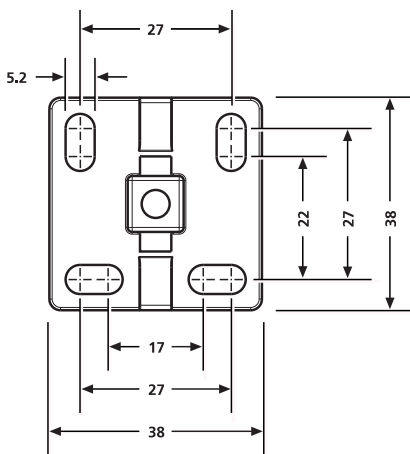
Helawrap HWBase und HWBaseA
