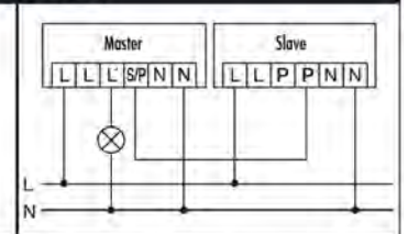
Master-Slave-Schaltung (es können max. 10 Slave-Geräte an ein Master-Gerät angeschlossen werden).
