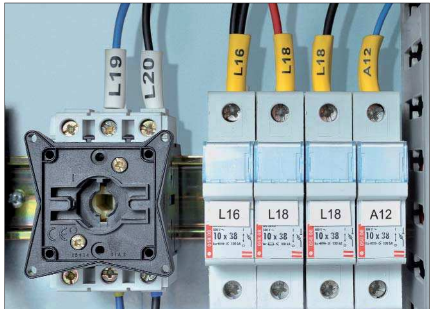
TULT - hochflexible Schrumpfschläuche in 5 Farben und 7 Größen.
