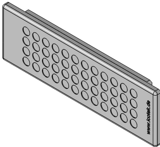
Kabeldurchführungplatte KEL-DP 24/48 48x Leitungsdurchmesser bis max 6,5 mm für Blechstärken von 1,5 bis 2,5 mm
