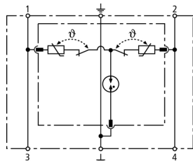
Prinzipialschaltbild DR M 2P 60
