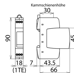
Maßbild DR M 2P 60
