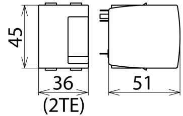
Maßbild DR MOD 4P 255
