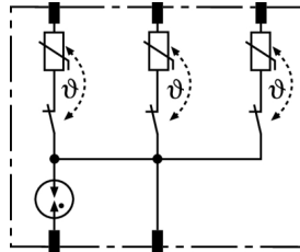
Prinzip Schaltbild DR MOD 4P 255
