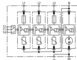
Prinzipialschaltbild DG M TT CI 275 FM
