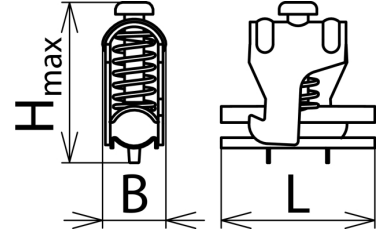
Maßbild SAK
