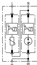
Prinzipschaltbild DG M TT 2P 385
