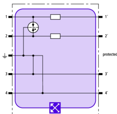
Prinzip Schaltbild BXT ML2 B 180
