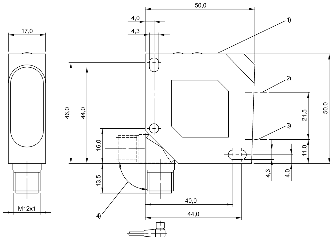
1) Anzeige- und Bedienfeld, 2) Optische Achse Sender, 3) Optische Achse Empfänger, 4) drehbar 270°
