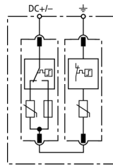
Prinzipialschaltbild DG S PV SCI 600
