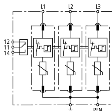
Prinzipschaltbild DG M TNC 440 FM
