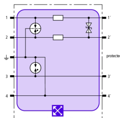
Principalschaltbild BXT ML2 BD DL S 15
