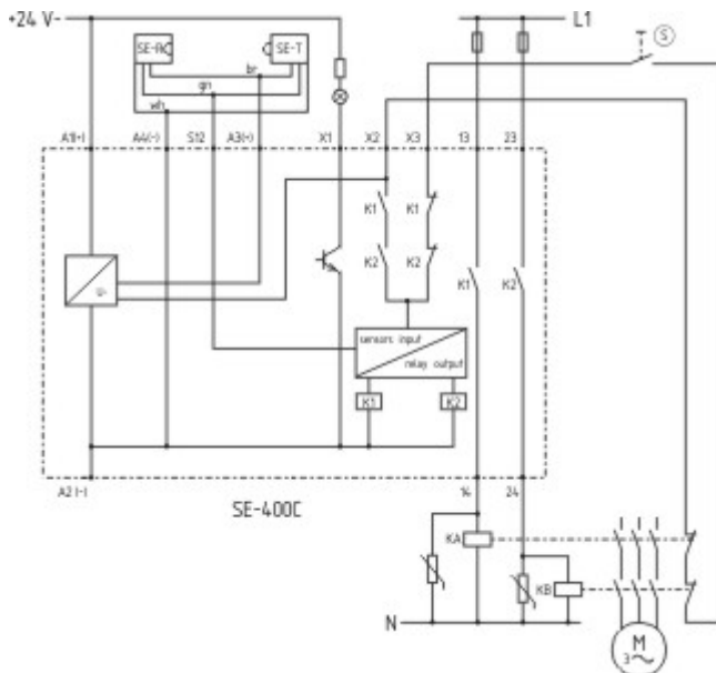
Schaltungsbeispiel
