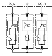
Prinzipialschaltbild DG M YPV SCI 600
