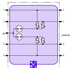
Prinzipschaltbild BXT ML4 MY 250
