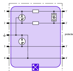
Prinzipschaltbild BXT ML2 BD HFS 5
