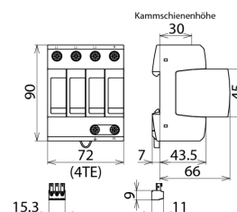
Maßbild DG M TNS CI 275 FM
