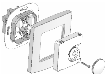
Regler 50 x 50 mit Alre-Rahmen Controller (50 x 50) with Alre type frame
