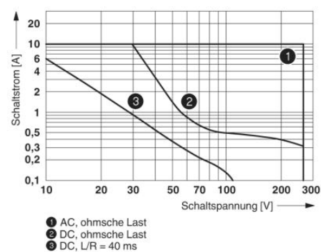
Abschaltleistung
