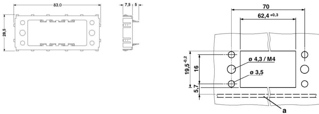
a - Leiterplatte
