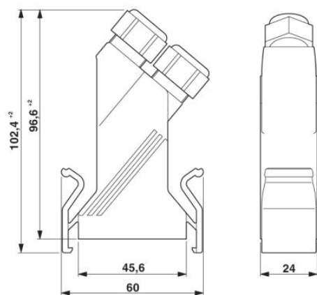
D-SUB Tüllengehäuse
