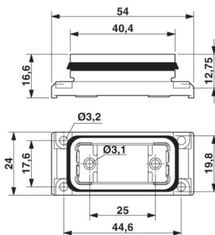
D-SUB Anbaurahmen
