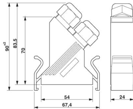
D-SUB Tüllengehäuse
