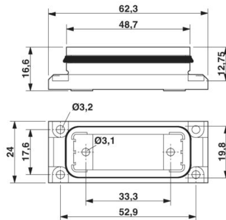
D-SUB Anbaurahmen
