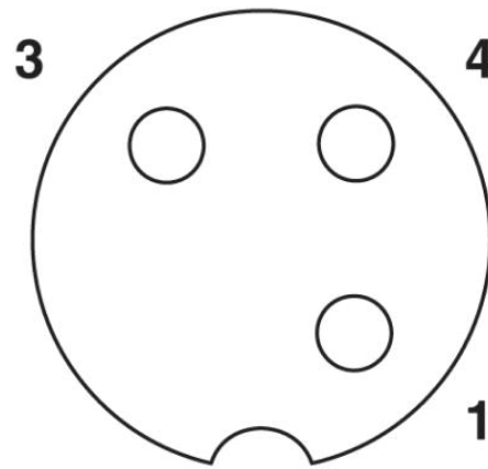
Polbild Buchse M12
