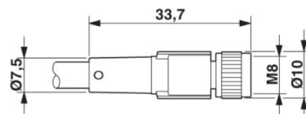
Buchse M8 x 1, gerade
