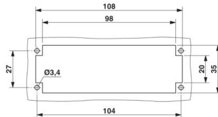
Montageausschnitt
