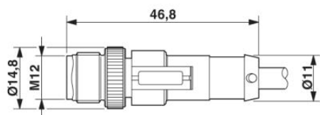
Stecker M12-SPEEDCON, gerade
