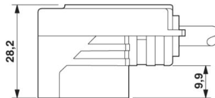
Ventilstecker, Bauform BI, Seitenansicht
