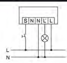
Standardbetrieb mit der zusätzlichen Ansteuerung durch Schließ-taster. Bei Bedarf kann das Licht durch den Taster manuell ein- bzw. ausgeschaltet werden.
