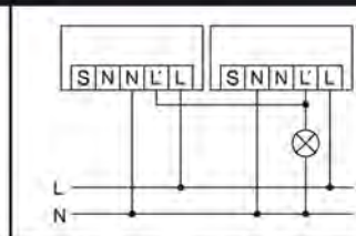
Parallelschaltung von max. 10 Geräten
