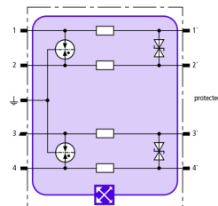
Prinzipschaltbild BXT ML4 BD 60
