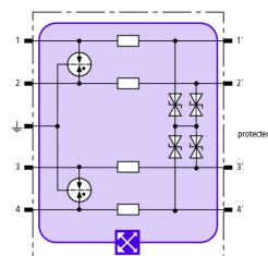
Prinzip Schaltbild BXT ML4 BC 5
