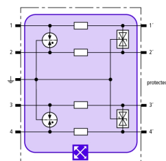
Prinzipialschaltbild BXT ML4 BE HF 5
