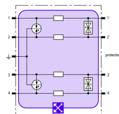
Prinzipschaltbild BXT ML4 BD HF 5
