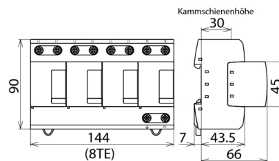
Maßbild DV M TT 255
