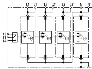
Prinzipialschaltbild DV M TT 255 FM
