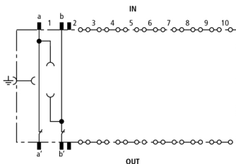
Principalschaltbild BM 10 DRL
