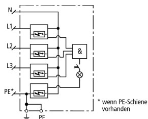
Principalschaltbild DV ZP TT 255
