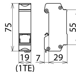
Maßbild DPA CLE RJ45B 48
