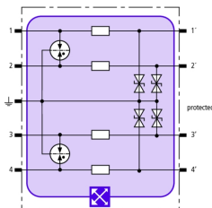
Prinzipschaltbild BXT ML4 BE 36
